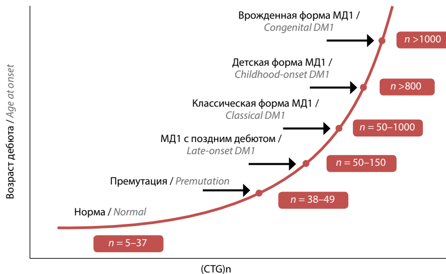
Рис. 1. При миотонической дистрофии 1-го типа (МД1) наблюдается нестабильная экспансия CTG-повторов. Количество CTG-повторов коррелирует с фенотипом заболевания Fig. 1. Unstable expansion of CTG repeats is observed in myotonic dystrophy type 1 (DM1). The number of CTG repeats correlates with the disease phenotype
